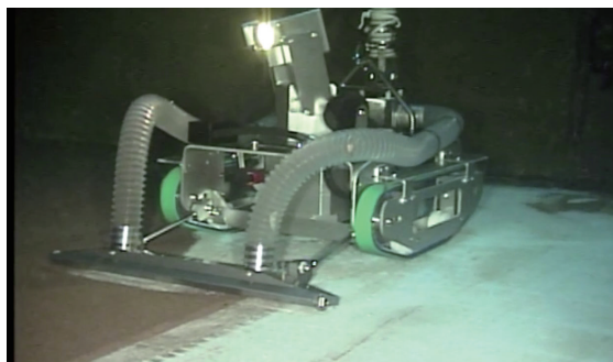
水中ロボット内部調査清掃状況
