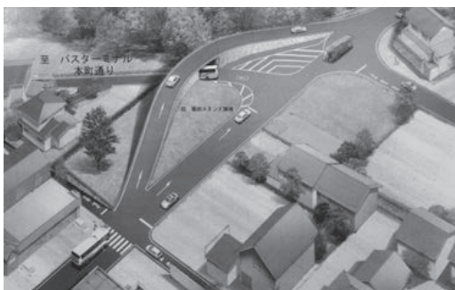
草津町独自の立体交差イメージ図
