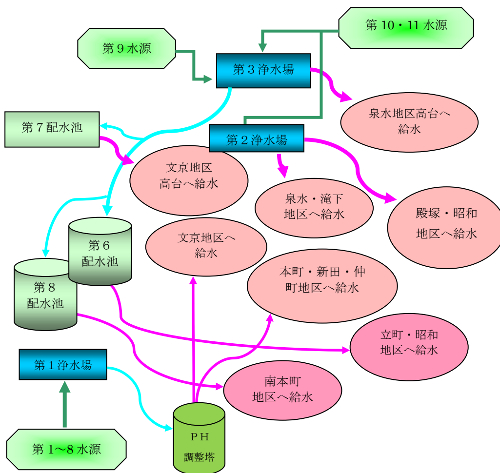
草津町上水道配水系統図
