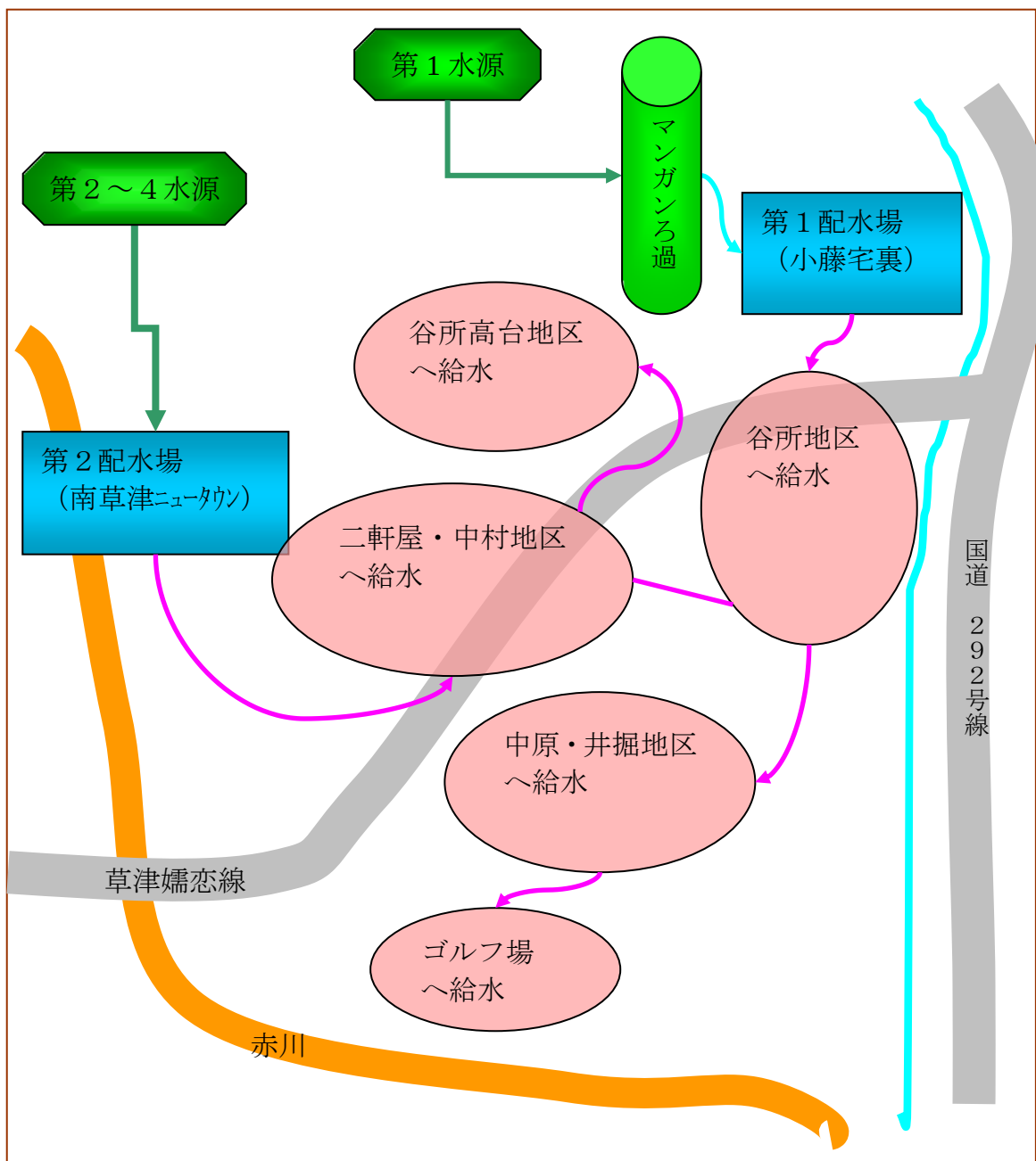
前口地区配水系統図
