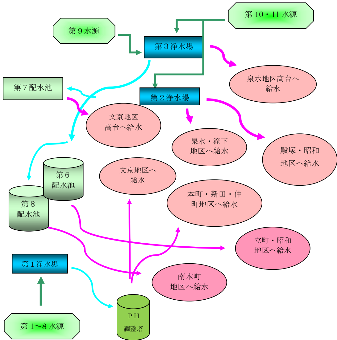
草津地区配水系統図
